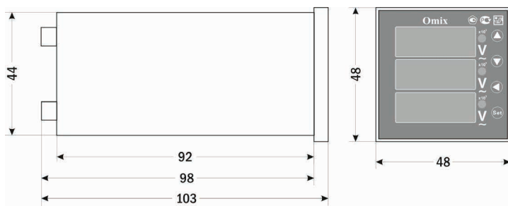
Рис. 3 – Размеры. Тип корпуса P44
